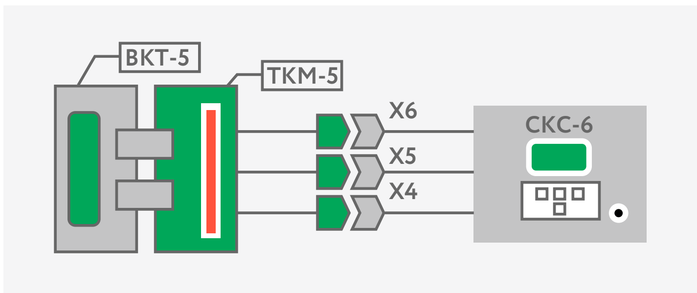
Рис. Б.2 Схема проверки ВКТ-5 с использованием СКС-6 и ТКМ-5 Разъемы X4...X6 (ТКМ-5) подключаются к одноименным разъемам стенда СКС6
