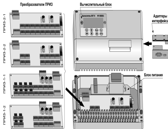
Рисунок 1 – Внешний вид составных частей контроллера
