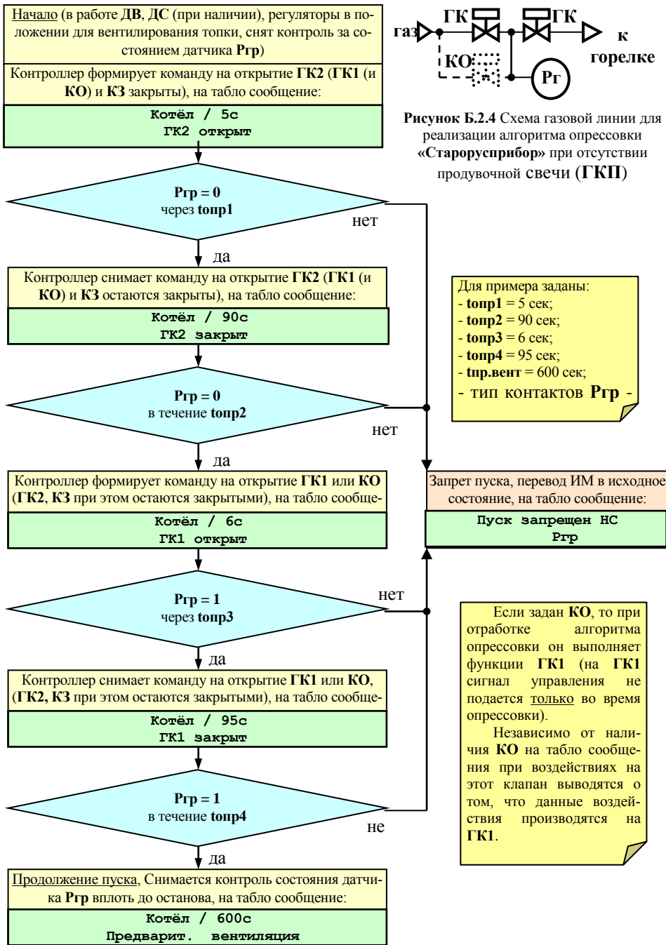
Рисунок Б.2.3 Блок-схема алгоритма варианта опрессовки «Старорусприбор» при отсутствии продувочной свечи (ГКП нет)
