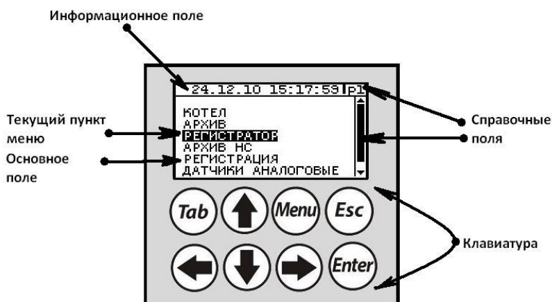
Рис.1.5.3.1 Табло контроллера
