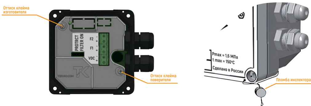
Рисунок 3. Места пломбирования
