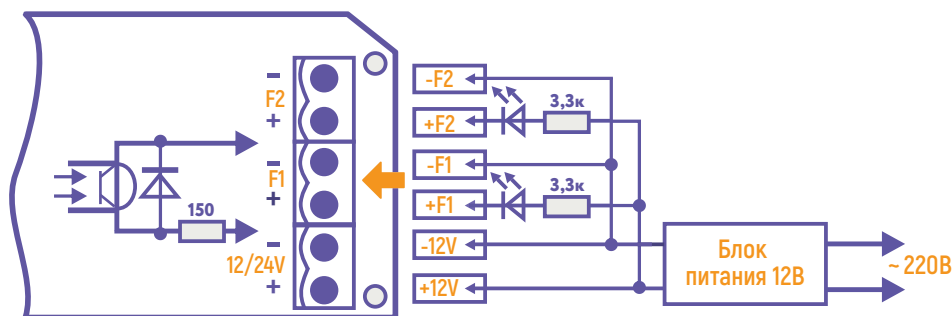
Рисунок 26. Контроль выходных сигналов 3523
