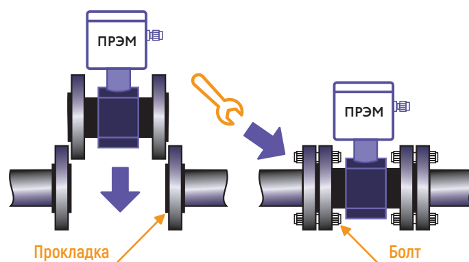
Рисунок 12. Способ установки ПРЭМ.
