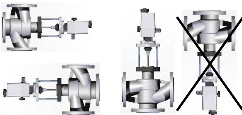
Рисунок А.4 Монтажные положения клапана с электроприводом REGADA ST 0; SAUTER AVF 234S F232. ПРИЛОЖЕНИЕ Б
