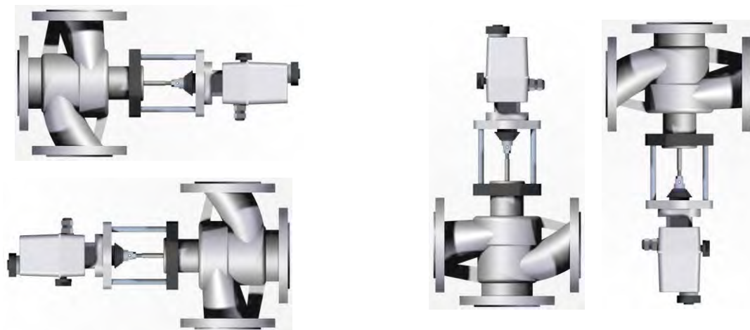
Рисунок А.3 Монтажные положения клапана с электроприводами ТЕПЛОСИЛА TSL-1600, -2200, REGADA: ST MINI, STR 0, ST 0.1, STR 0.1.
