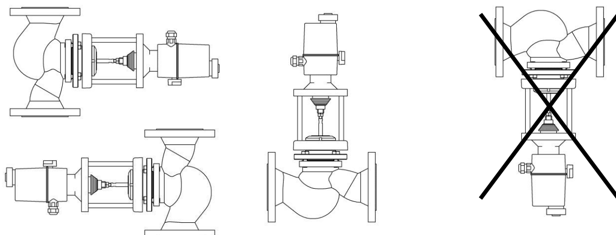
Рисунок А.5 Монтажные положения клапана с электроприводом REGADA ST 0; SAUTER AVF 234S F232.
