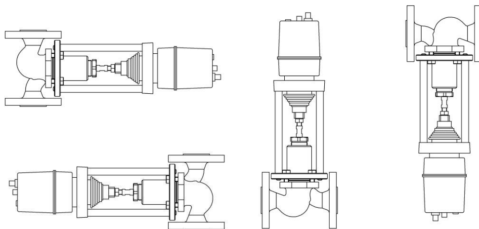
Рисунок А.4 Монтажные положения клапана с электроприводами TSL-1600, -2200 REGADA: ST MINI, STR 0, ST 0.1, STR 0.1, ST 1, STR 1.
